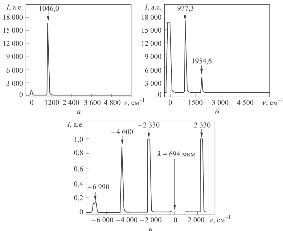
Рис. 8. Спектры ВКР света на полносимметричных модах в монокристалле кальцита ( а ), в порошке органического соединения РОРОР ( б ) и жидком азоте ( в )
