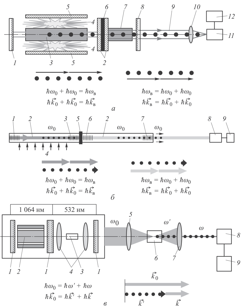
Рис. 13 (начало). Предлагаемые схемы для осуществления различных процессов фотон-бозонной конверсии в материальных средах: a — для фотон-парафотонной конверсии в резонаторе рубинового лазера (1, 2, 8 — зеркала; 3 — активный элемент лазера на рубине; 4 — лампы накачки; 5 — отражатель; 6 — непрозрачная стенка; 7 — рубин; 9 — излучение; 10 — линза; 11, 12 — детекторы); б — для фотон-парафотонной конверсии в резонаторе эрбиевого лазера (1, 3, 6, 7 — брэгговские зеркала; 2 — кварцевый световод, легированный эрбием; 4 — накачка; 5 — непрозрачная стенка; 8, 9 — детекторы); в — для парафотонного рассеяния света в щелочно-галогидных кристаллах (1 — зеркала; 2 — активный элемент; 3 — нелинейный кристалл; 4, 5, 7 — линзы; 6 — щелочно-галогидный кристалл; 8, 9 — детекторы)
