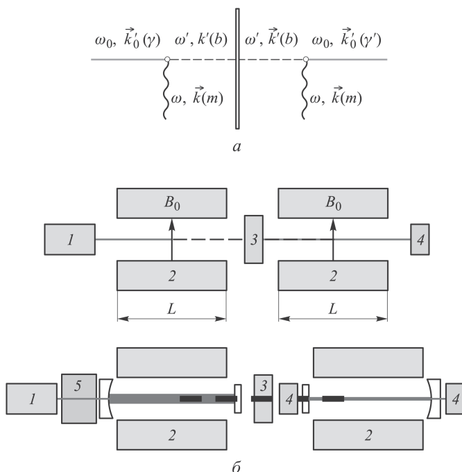
Рис. 12. Принципиальные схемы для осуществления фотон-аксионной конверсии в магнитном поле без дополнительного резонатора (а) и с интерферометром Фабри – Перо (б):
