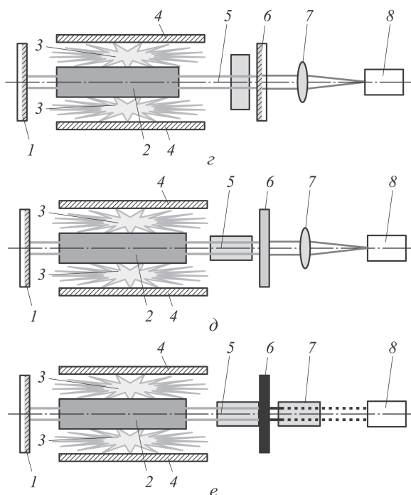
Рис. 13 (окончание). а — для регистрации инфракрасного излучения при ВКР на поперечных поляритонах в кристалле ниобата лития, оптическая ось которого перпендикулярна направлению распространения возбуждающего излучения ( 1 — зеркало; 2 — активный элемент; 3 — лампы; 4 — отражатель; 5 — кристалл; 7 — линза; 8 — детектор); б — для регистрации инфракрасного излучения при ВКР на продольных поляритонах в кристалле ниобата лития, оптическая ось которого совпадает с направлением распространения возбуждающего излучения ( 1 — зеркало; 2 — активный элемент; 3 — лампы; 4 — экран; 5 — кристалл; 6 — непрозрачная стенка; 7 — линза; 8 — детектор); в — для регистрации инфракрасного излучения при ВКР на продольных поляритонах в кристалле ниобата лития, оптическая ось которого совпадает с направлением распространения возбуждающего излучения ( 1 — зеркало; 2 — активный элемент; 3 — лампы; 4 — экран; 5 , 7 — кристаллы; 6 — непрозрачная стенка; 8 — детектор)
